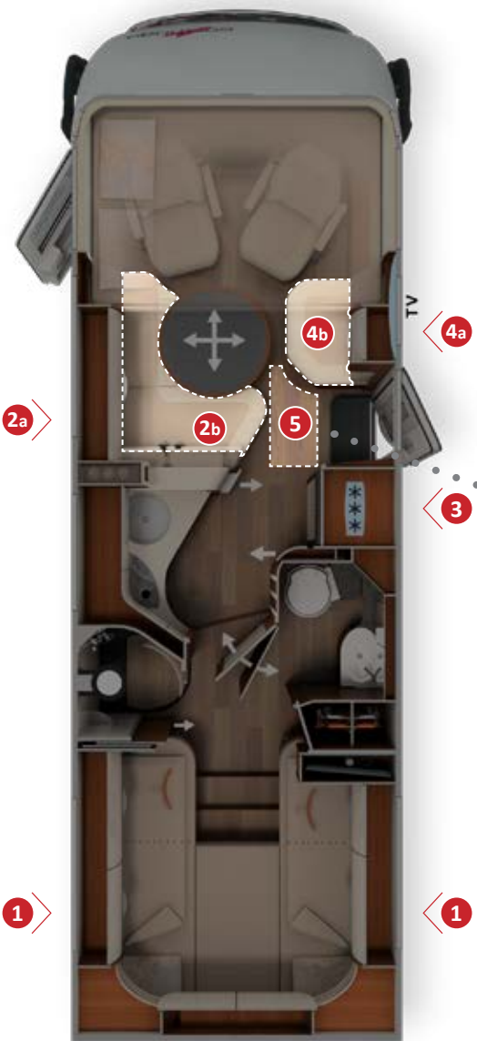
Rollergarage mit großer Innenhöhe durch tiefe Absenkung, beidseitiger Zugang über zwei große Rollergaragentüren auf Fahrer- und Beifahrerseite
